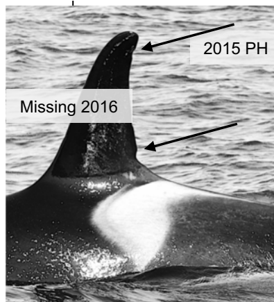
AD 5 (<1961) Elli
